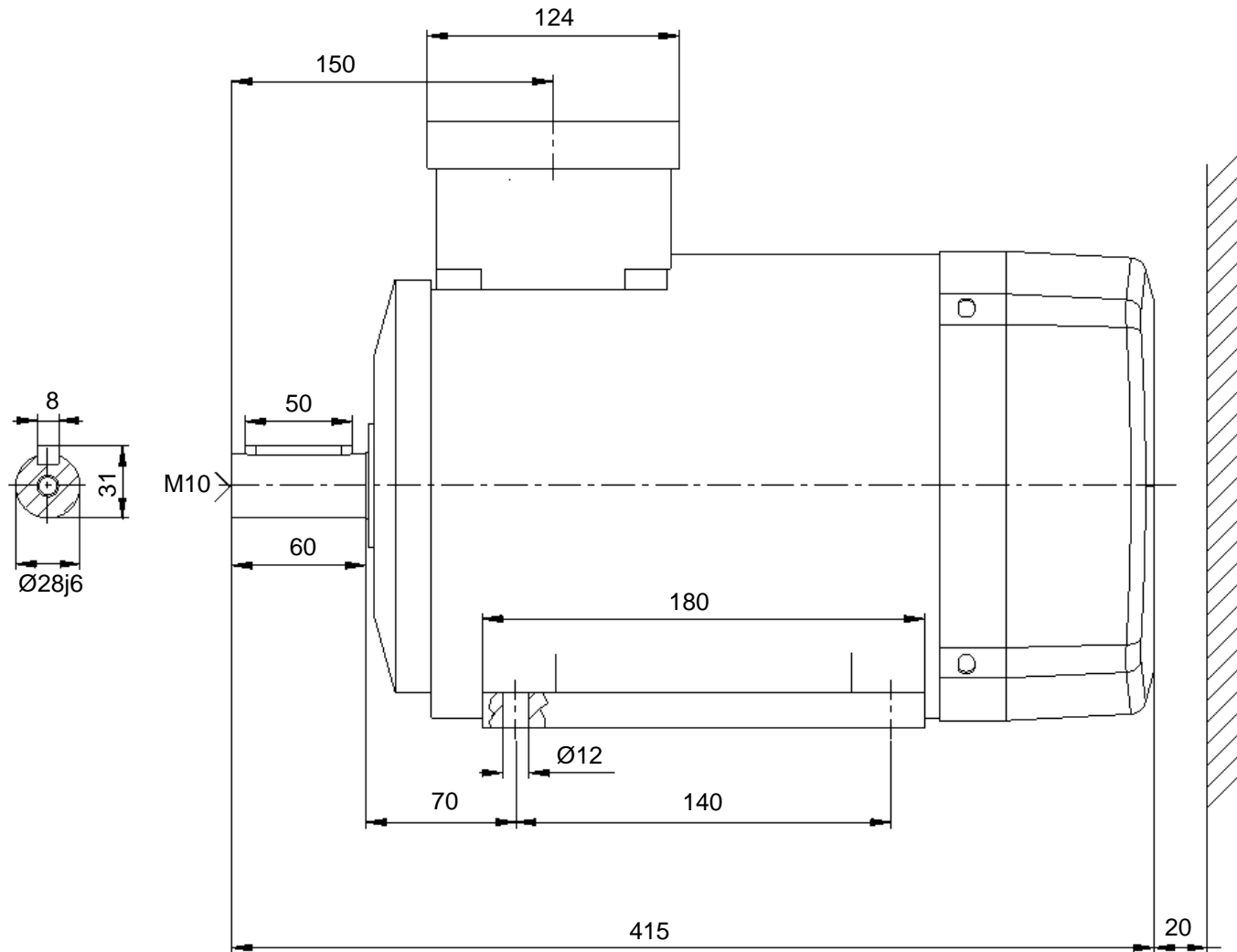
Maßblatt - #713195 - KDG2C 112 M 2 KT FL IE3 in Angebot An161836 Position 1 Kabelverschraubung: 2x M25x1,5
