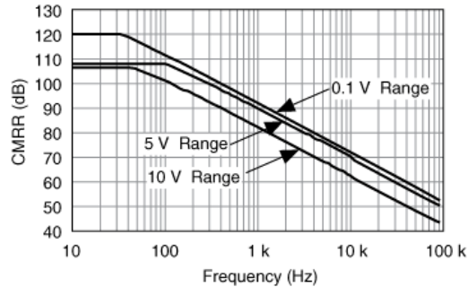
AI <0..79> CMRR
