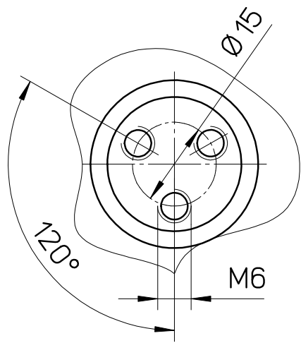
Particolare foratura albero
