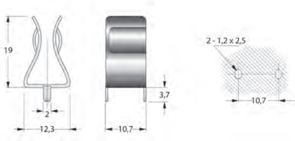
PINZE PER FUSIBILI 10x38 0900502 FUSE CLIPS FOR FUSES 10x38 0900502
