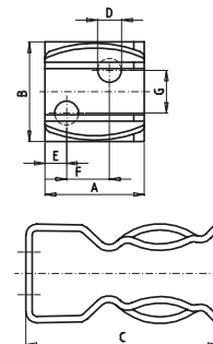
PINZE PER FUSIBILI 22x58 0900508 FUSE CLIPS FOR FUSES 22x58 0900508
