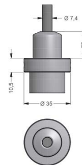
Kabelausgang mit Belüftungsschlauch (IP 68) 6 (auf Anfrage)
