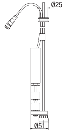
Fig. 3: Type SL-2
