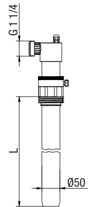
Fig. 12: Type SDL-2 DN15
