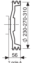
Puleggia Pulley Polea Poulie Keilriemenscheibe
