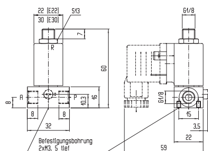
Ausführung mit Gewindeanschluss G 1/8
